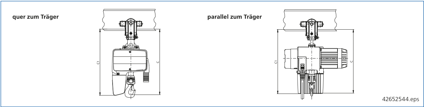
Maßtabelle Kettenzug DC-Pro mit Fahrwerk CF 5
