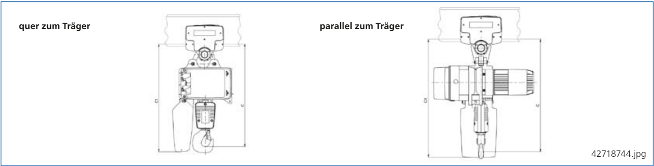
Maßtabelle Kettenzug DC-Pro 16 und 25 mit Fahrwerk U 22, U 34, RU 56
