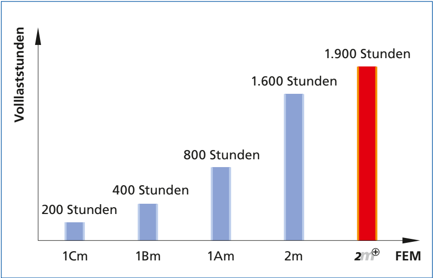
Volllaststunden-Nutzungsdauer
