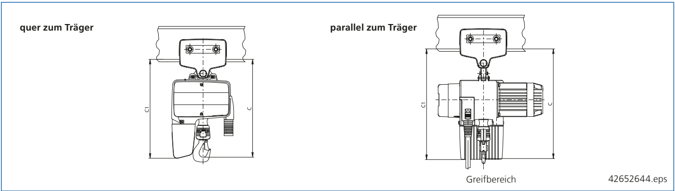
Maßtabelle Kettenzug DC-Pro 1–10 mit Fahrwerk U 11, U 22 oder U 34
